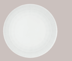
MAR HOTEL 21130428 Prato Marcador Redondo 33 Round Charger Plate 33 Plato Presentación Redondo 33 Assiette de Présentation Ronde 33 △ 1170 gr A 23 mm Ø 330 mm △ 2 1/2 lbs H 3/8" Ø 13"
